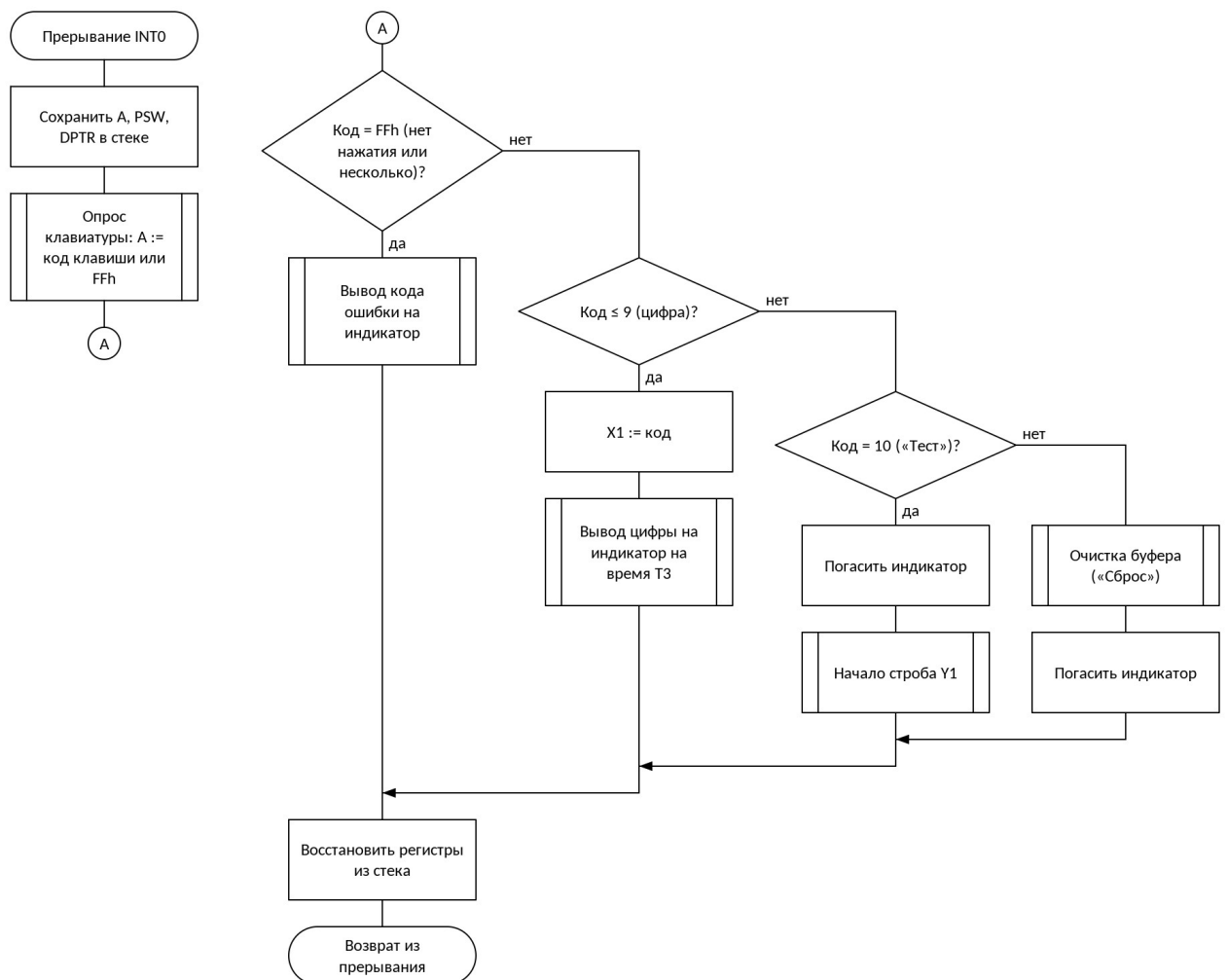
Рисунок 4 — Схема алгоритма: Обработчик прерывания INT0: реакция на клавишу
