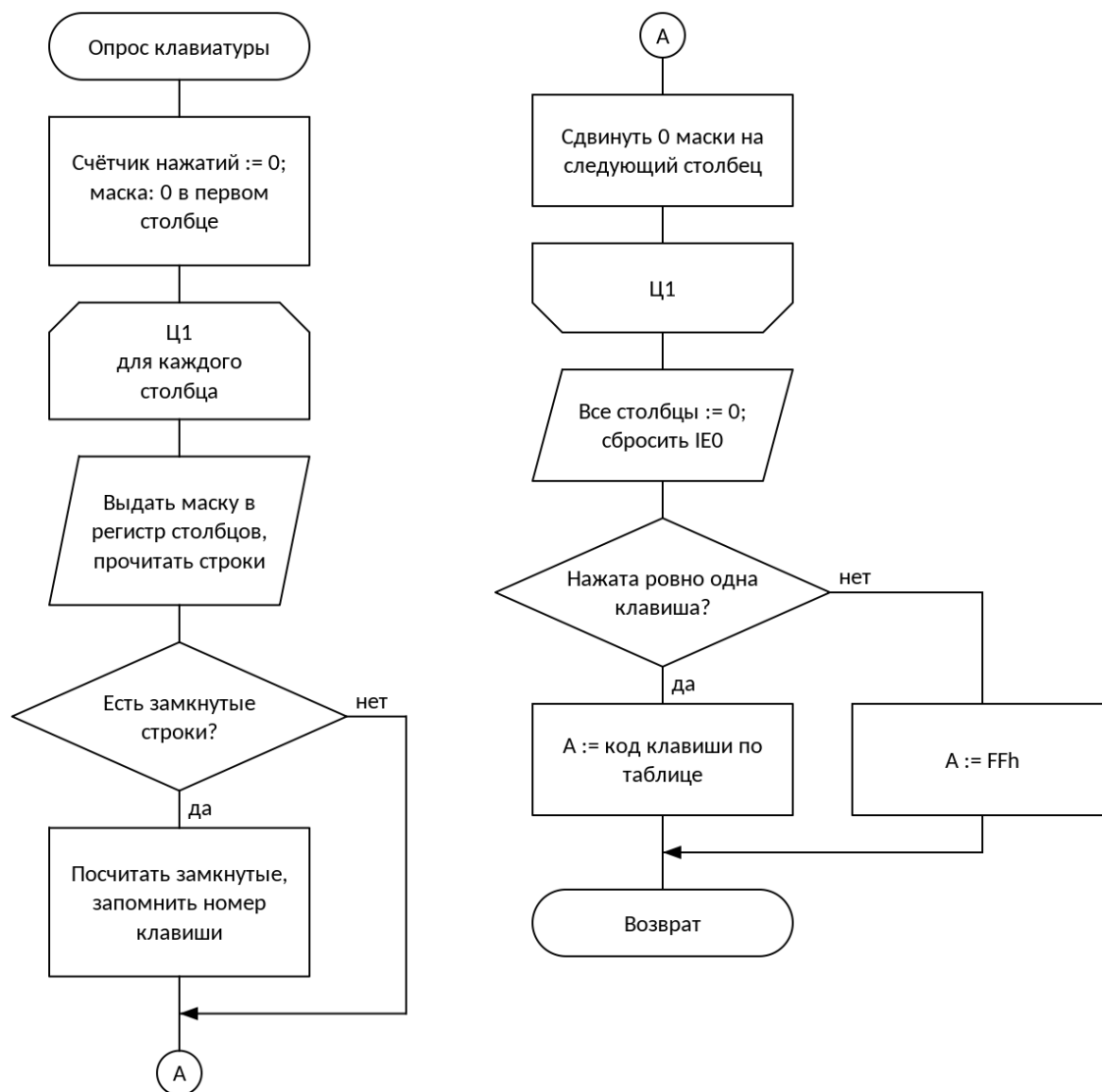
Рисунок 3 — Схема алгоритма: Опрос клавиатуры (обработчик INT0)
