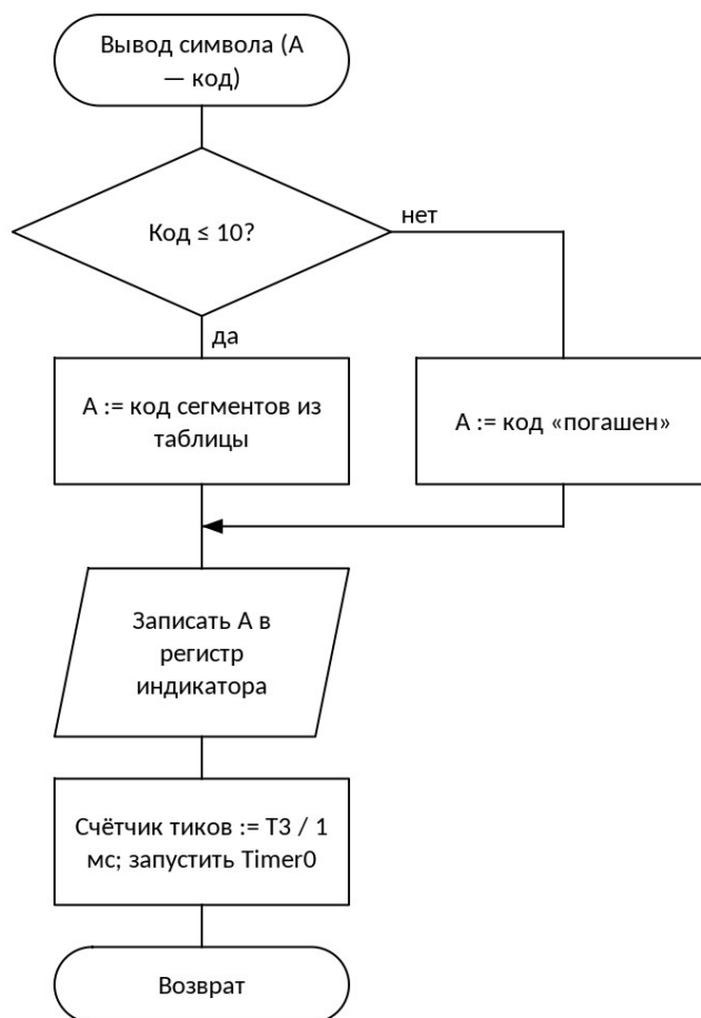
Рисунок 9 — Схема алгоритма: Вывод символа на индикатор
