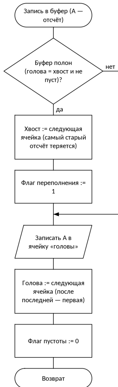
Рисунок 5 — Схема алгоритма: Запись отсчёта в кольцевой буфер
